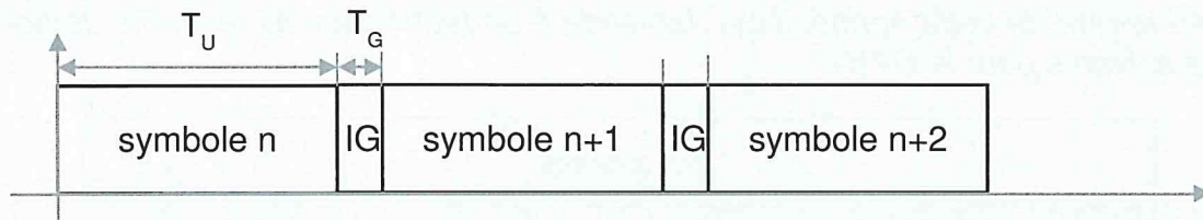
Figure 4 - Répartition temporelle des symboles
